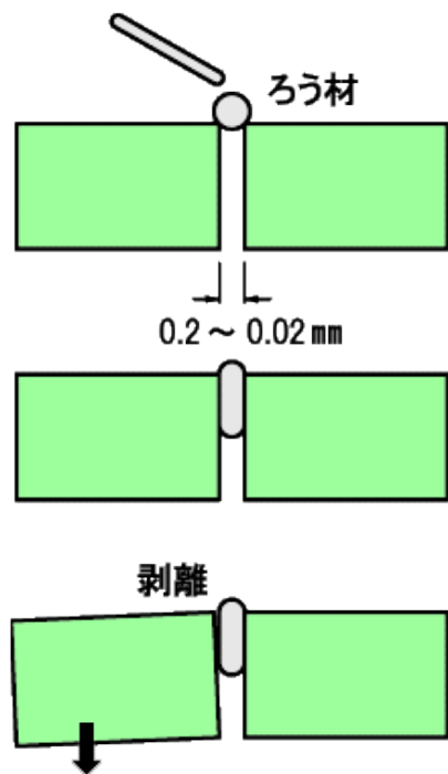
図1. 非加熱母材にろう付した場合
