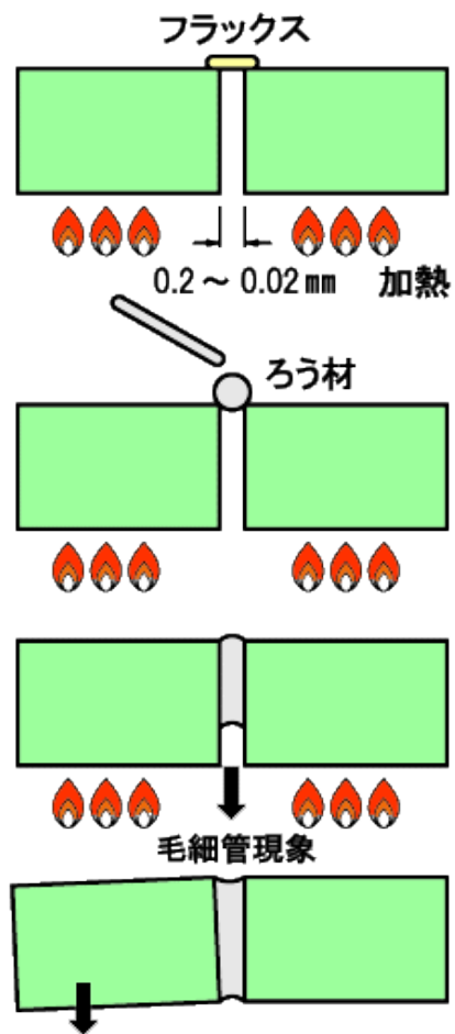
図2. 母材を加熱しろう付した場合
